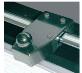
Chariot de coupe avec lame rotative auto-affutante
